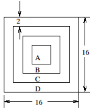
Figure 14: 16 \times 16 subarea
